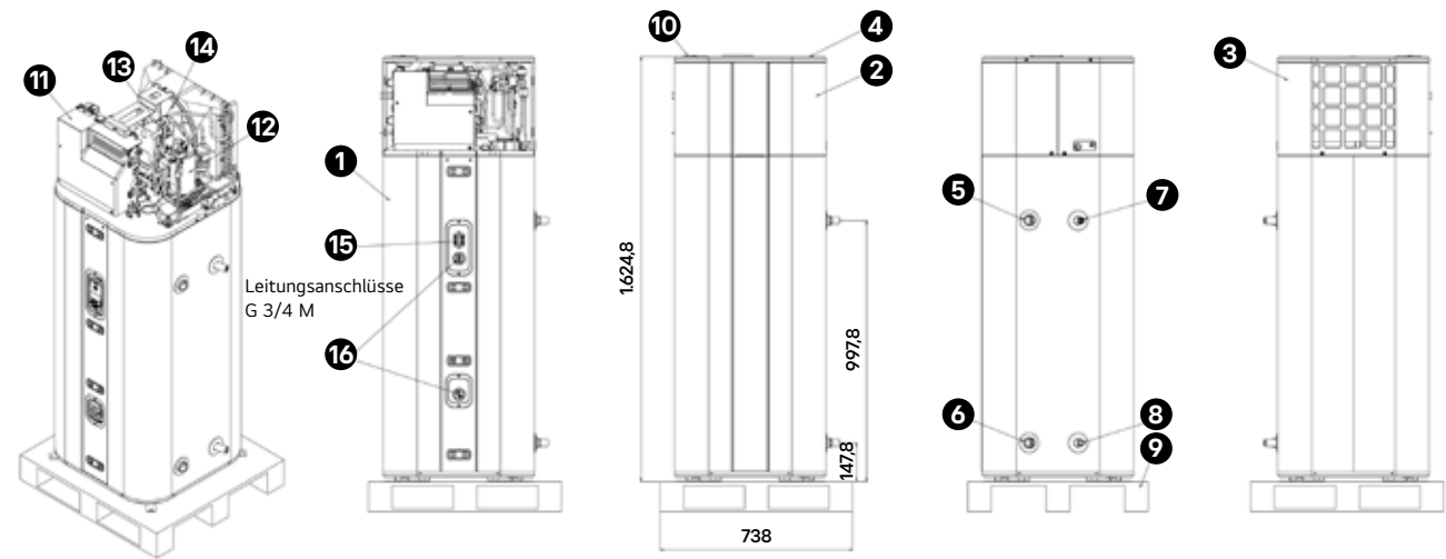
3D-Innenansicht
